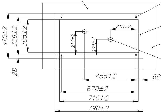
Рисунок А.1 Колонка топливораздаточная "Топаз-421-XX-X000/00"
